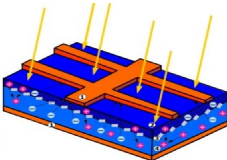
Rysunek 5 Budowa i sposób działania ogniw fotowoltaicznych
