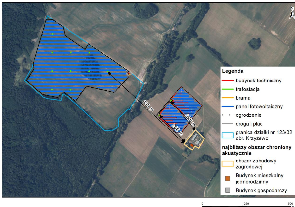
Rysunek 24 Odległości źródeł dźwięku od zabudowy mieszkaniowej na farmie fotowoltaicznej w wariantcie alternatywnym oraz na farmach na działkach 170/15 oraz 2/3 obr. Krzyżewo
