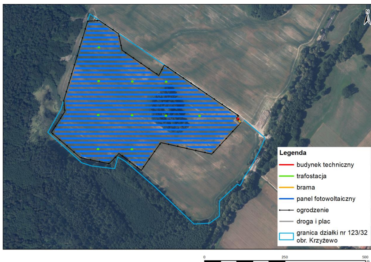
Rysunek 22 Rozmieszczenie infrastruktury na farmie w wariantcie alternatywnym
